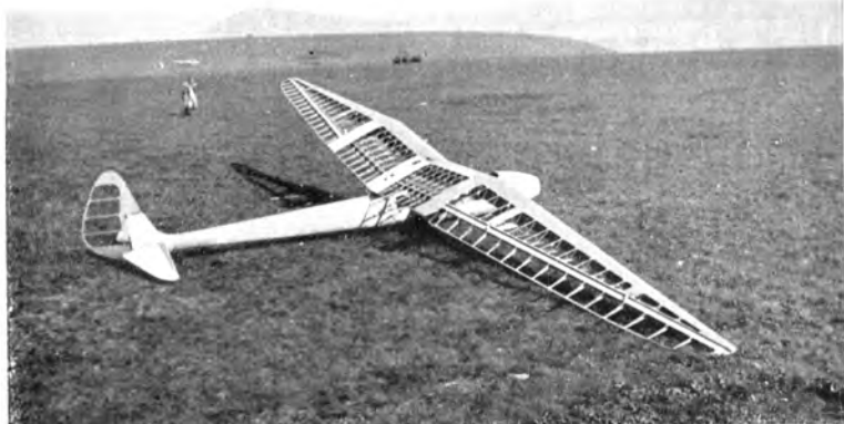
Rohbau des „Condor I“ auf der Wäckerkuppe
