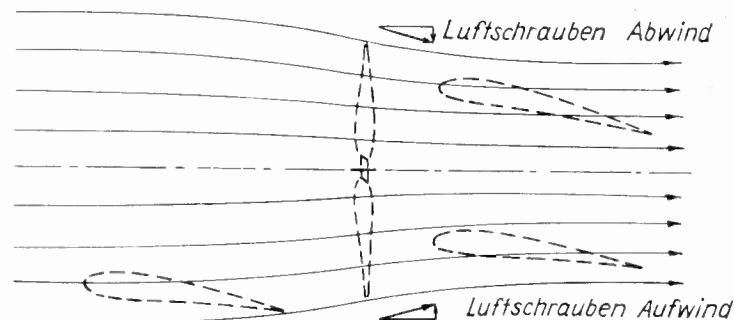
Abb. 45. Die Luftschaubenströmung und ihre Wirkung auf den Flügel in verschiedenen Stellungen.
