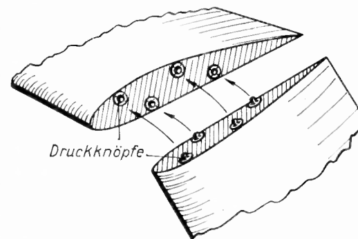
Abb. 64a. Flügelanlüsse durch Druckknöpfe nach Gentsch.
