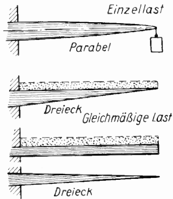
Abb. 53. Nach dem Ende verjüngte Freitrager bei verschiedener Lastverteilung.
