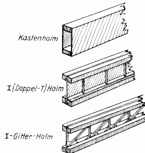
Abb. 51. Verschiedene Holmbauweisen.
