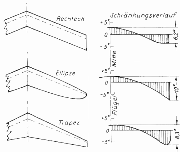
Abb. 21. Der günstige Schränkungverlauf bei stabilen Pfeilflügeln mit verschiedener Umrißform. (Die gleichen wie Abb. 14.)
