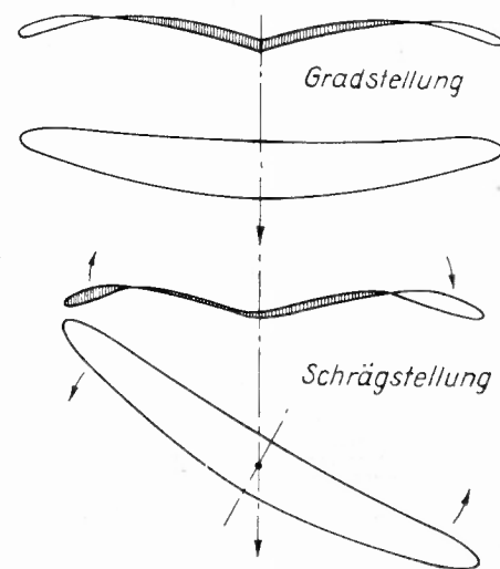
Abb. 19. Quer- und Richtungsstabilität des Fasnirflügels.
