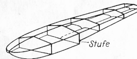
Abb. 82. Schwimmer.
