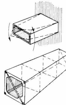
Abb. 54. Der torsionssteife Kasten (Bierkan-Rumpf) muß allseitig geschlossen sein.
