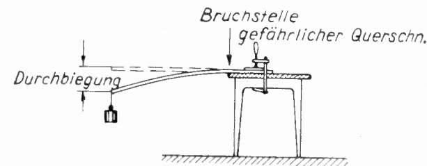
Abb. 48. Einfacher Biegeversuch.
