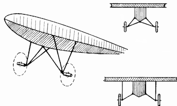
Abb. 79. Achslose Fahrwerkankordnungen.
