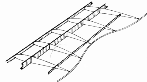
Abb. 26. Richtige Profiländerung in der Gegend des Flügelausschnittes.
