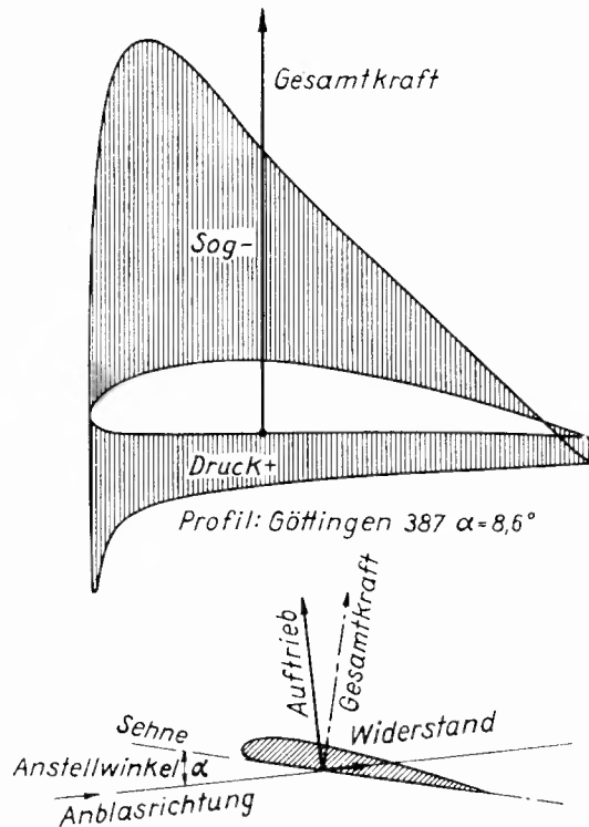
Abb. 9. Druckverteilung am Profil, Anstellwinkel und Luftkräfte.
