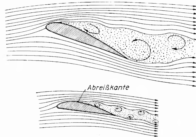
Abb. 10. Abgerissene Flügelströmung.
