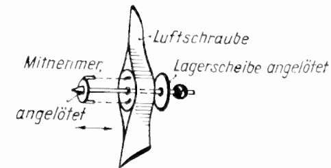
Abb. 38. Kuppelungseinrichtung an der Luftschraubenlagerung.
