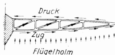
Abb. 46c. Kräfte in einem Fachwerkhalm.
