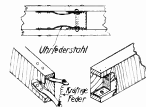
Abb. 64b. Lösbare Holmverbindung mit Stahlfederung.
