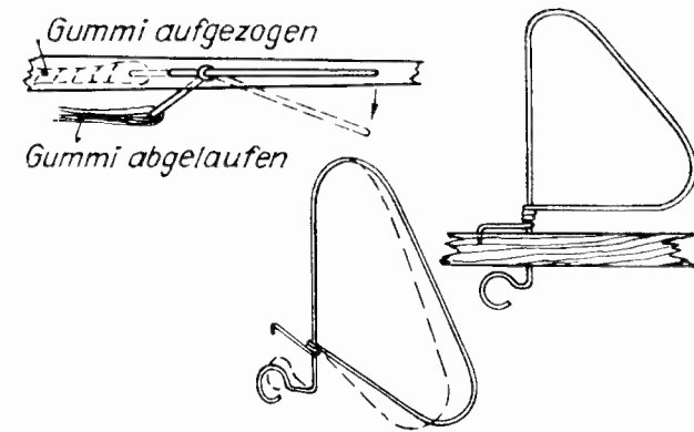
Abb. 75. Stahldraht-Seitenleitwerk mit automatischem Motor-Drehmomentausgleich.
