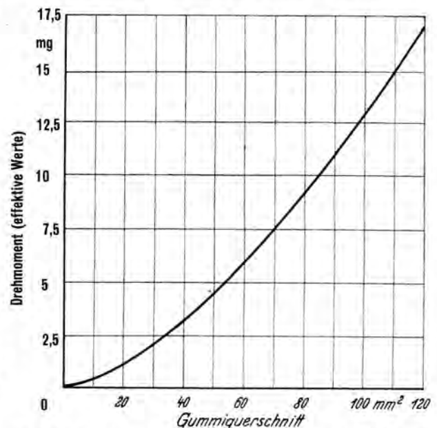
Abb. 3. Effektivwerte des Drehmomentes in Abhängigkeit vom Gummiquerschnitt
