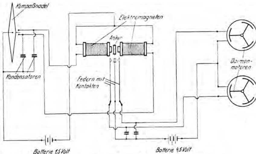
Abb. 2. Schaltschema einer Kompaßsteuerung mit Zwischenrelais
