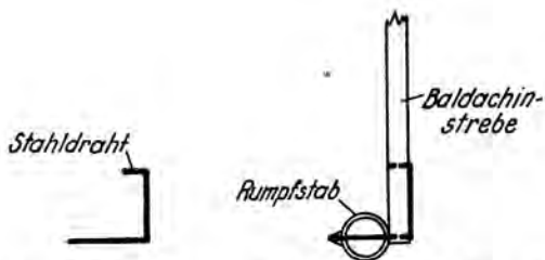
Abb. 3. Befestigung einer Baldachinstrebe am Rumpfstab
