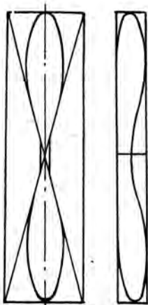
Abb. 5. Bemessung der nabennahen Teile der Luftschraube
