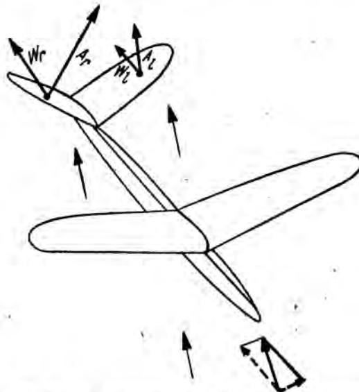
Abb. 9. Wirkung des V-Leitwerkes bei schiefer Querlage im Gleitflug
