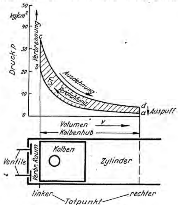
Abb. 3. Diagramm des Selbstzündermotors
