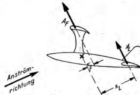
Abb. 15. Kräftespiel beim Kraftflug
