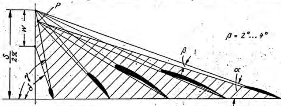
Abb. 1. Die Steigungsverkleinerung am Luftschraubenstrahl
