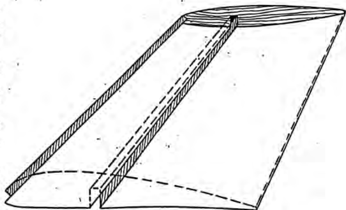
Abb. 3. Holzblock für einen sich verjüngenden Flügel
