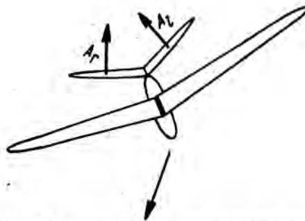
Abb. 9. Wirkung des V-Leitwerkes bei schiefer Querlage im Gleitflug
