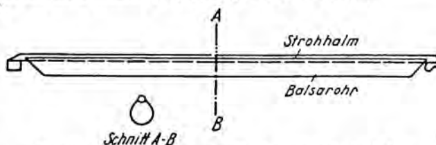
Abb. 2. Vollrumpfbauweise für das Drehflügel-Hallenflugmodell von Scheiffele
