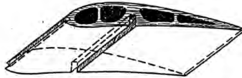
Abb. 2. Der geteilte Holzblock mit den ausgearbeiteten Erleichterungsaussparungen
