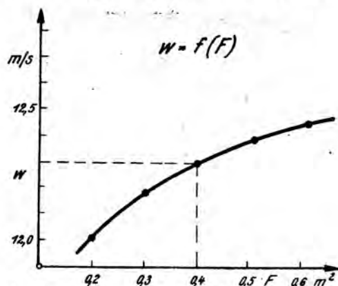
Abb. 2. Steigleistung als Funktion der Flügelfläche
