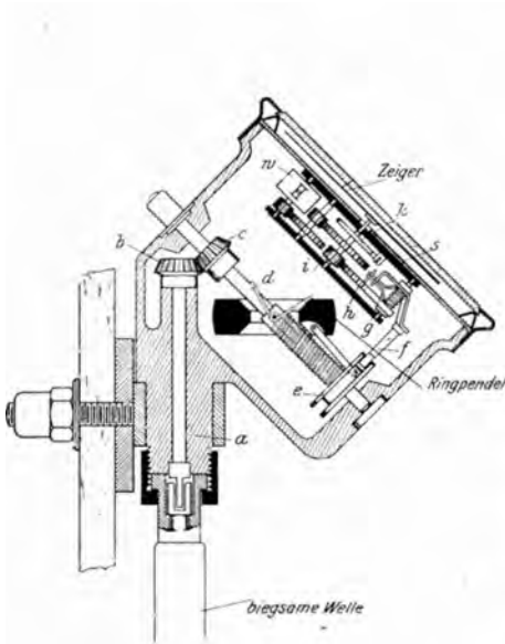
Abb. 1. Schema eines Drehzahlmessers mit Fliehpendel (Morell).
