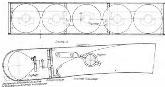
Abb. 296. Rampenbeleuchtung nach Dr. Neuber.
