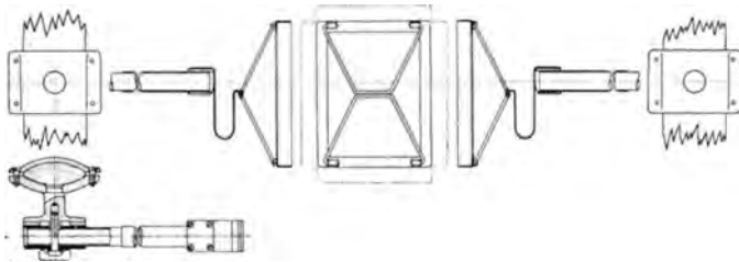
Abb. 141. Befestigungsvorrichtung für Höhenschreiber nach Oppermann (Goerz).
