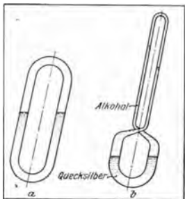
Abb. 172. a) gewöhnliches U-Rohr; b) U-Rohr nach Dr. Neuber.
