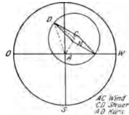
Abb. 228. Schema des Reisekompasses nach Bennewitz.
