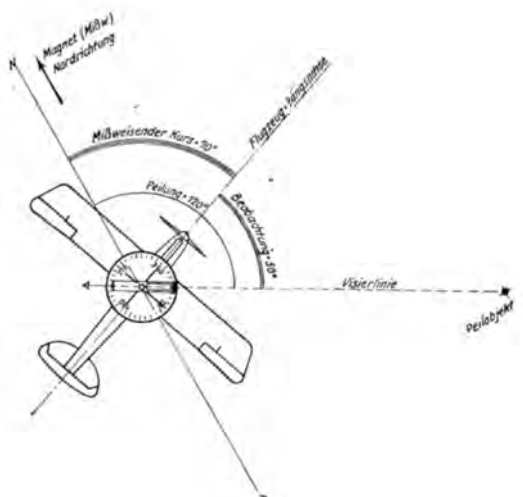
Abb. 236. Anwendung der Peilscheibe.
