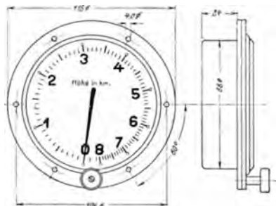
Abb. 95. Normalhöhenmesser (mittlerer Typ).
