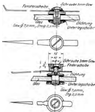
Abb. 209. Normalien des Kurszeigers.
