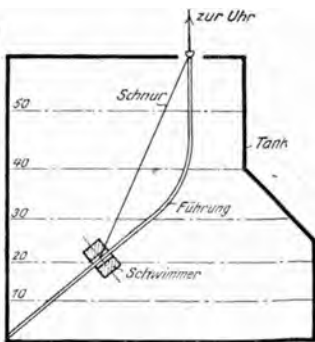
Abb. 45. Lineare Schwimmerführung.
