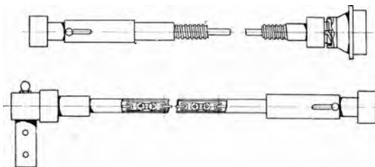
Abb. 31. Biegsame Wellen (Morell).
