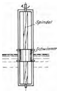
Abb. 41. Benzinuhr mit Spindel.
