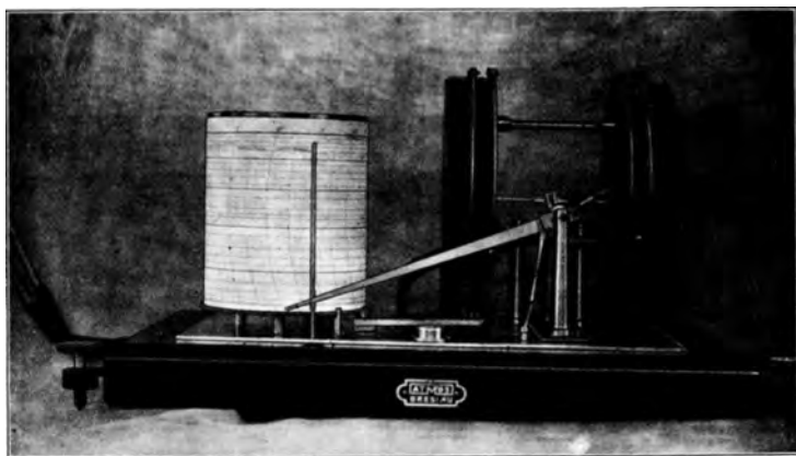
Abb. 272. Staudruck-Fahrtsschreiber (Atmos).
