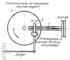
Abb. 15. Schema eines Drehzahlmessers mit Reibrad (Behrens).
