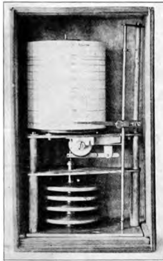
Abb. 123. Höhenschreiber (v. d. Borne).
