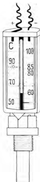
Abb. 68. Kühlwasserthermometer (Jahn).
