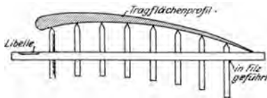
Abb. 379. Verspannungsmesser nach Bennewitz.
