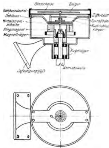
Abb. 11. Schema eines Wirbelstromdrehzahlmessers („O. S.“).
