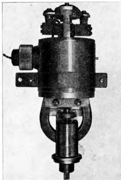
Abb. 24. Fern-drehzahlmesser (Horn). Geber.
