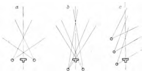
Abb. 302. Verteilung der Lichtquellen für Landbahnbeleuchtung.
