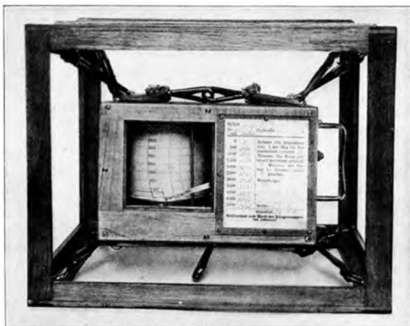
Abb. 140. Abfederung bei stehenden Höhenschreibern
