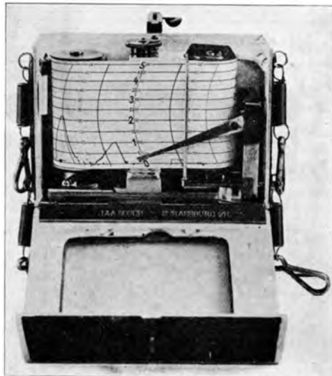
Abb. 124. Höhenschreiber (Bosch).
