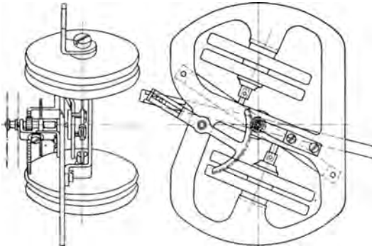
Abb. 86. Hebelwerk (Goerz).
