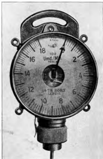
Abb. 23. Ferndrehzahlmesser (Horn). Anzeiger.
