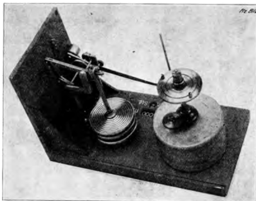
Abb. 113. Höhenschreiberwerk (Goertz).
