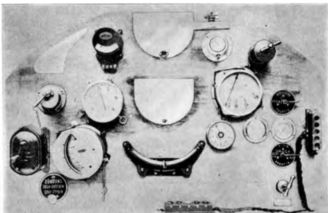
Abb. 384. Fehlerhafter Einbau.
