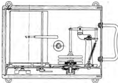
Abb. 107 Höhengschreiber (Goerz).
