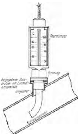
Abb. 69. Einbau-Normalstutzen.
