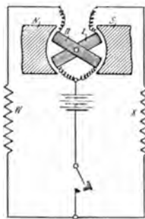
Abb. 74. Schema der Temperaturmessung mittels Differentialgalvanometers.
