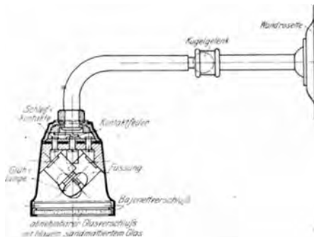
Abb. 288. Soffittenlampe (Dr. Schneider).
