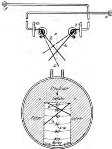
Abb. 187. (a und b) Staudruckkurvenmesser nach Bennewitz.
