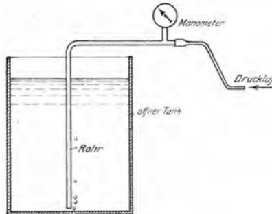
Abb. 47. Benzinuhr mit Druckluft nach Hirth.
