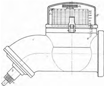
Abb. 8. Aufriß des Drehzahlstreibers (Horn).
