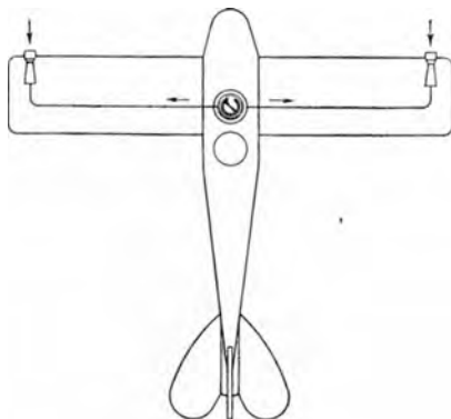
Abb. 186. Prinzip eines Staudruckkurvenmessers.
