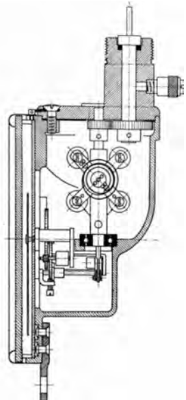
Abb. 2. Drehzahlmesser mit Doppelpendel (Bundschuh)-
