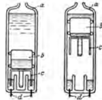
Abb. 144. Dichtemessung durch Taucher.
