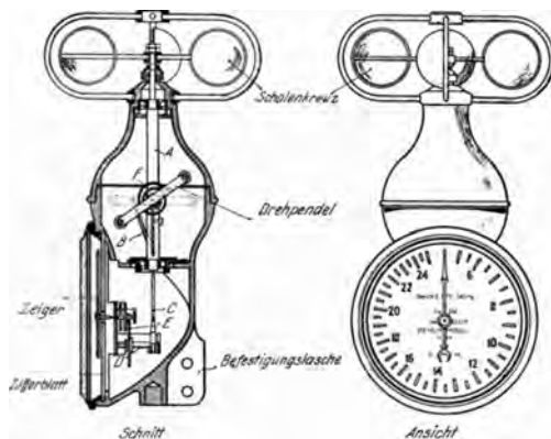
Abb. 246 u. 247. Schema des Schalenkreuz-Fahrtmessers (Morell).
