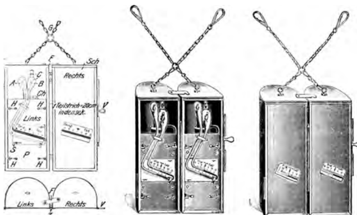
Abb. 158. Variometer „Bestelmeier“ (Hase).
