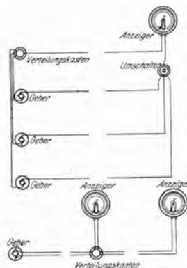
Abb. 29. Schaltschema für Mehrfachdrehzahlmesser.
