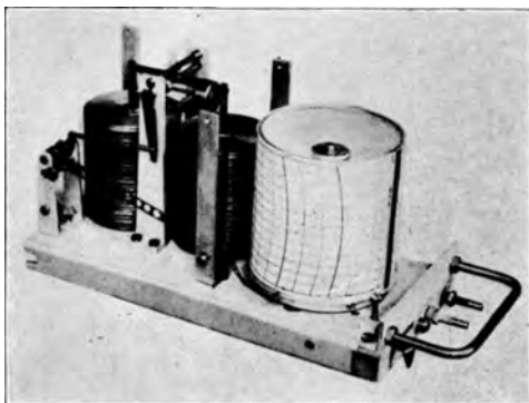
Abb. 271. Staudruck-Fahrtsschreiber (A. E.-G.).
