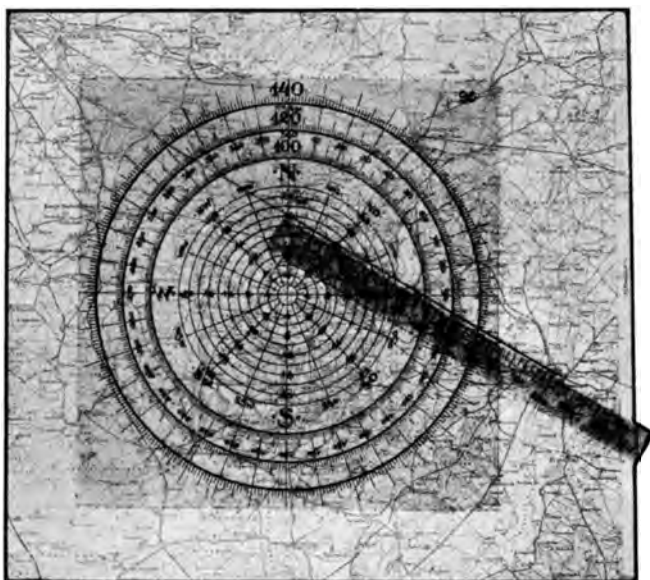
Abb. 225. Anwendung des Winddreiecks (Wichmann).
