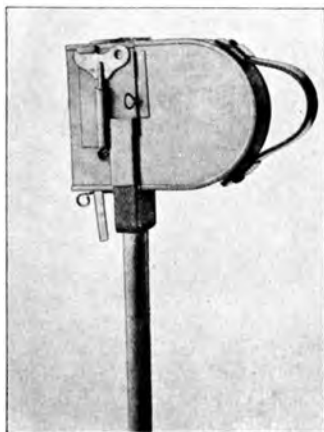
Abb. 307. Magnesiumfackel (Boehm).
