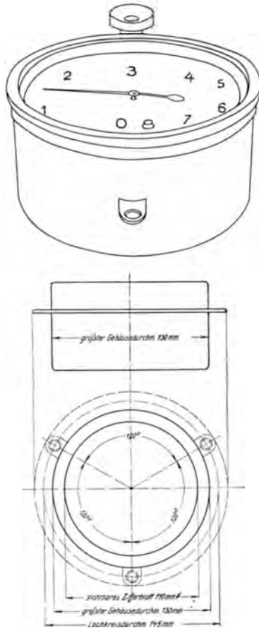
Abb. 94. Normalhöhenmesser (großer Typ).
