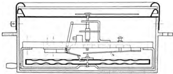
Abb. 263. Staudruck-Fahrtmesser mit Ausgleichsfeder a (Eckardt).
