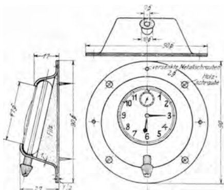
Abb. 376. Gehäuse für Borduhren.
