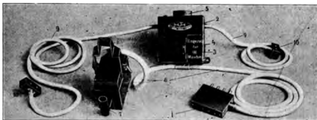
Abb. 349. Heizleitung in Verbindung mit F. T.-Taster.
