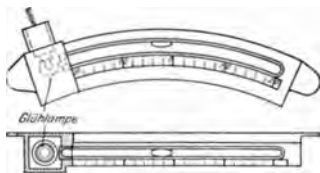
Abb. 167. Libelle als Neigungsmesser.
