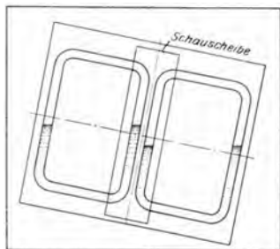
Abb. 174. Neigungsmesser (Weise).
