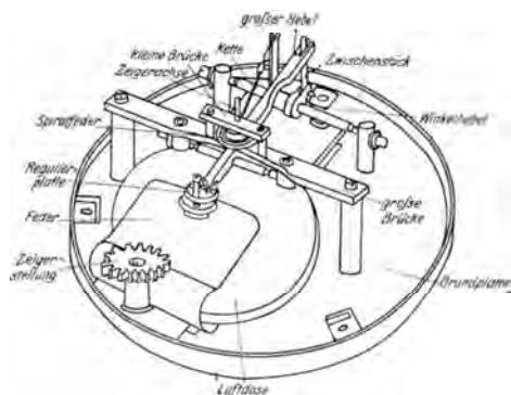
Abb. 88. Hebelwerk (Kröplin).
