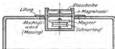
Abb. 40. Magnetische Übertragung der Anzeige.
