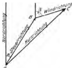
Abb. 227. Winddreieck.
