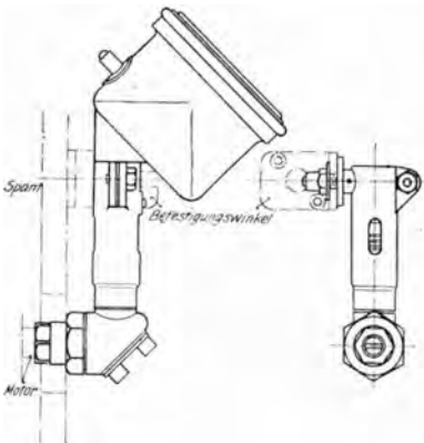
Abb. 33. Anschlußstück (Morell).
