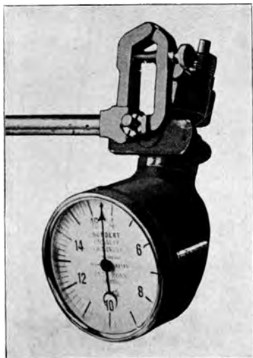
Abb. 6. Drehzahlmesser mit oberem Antrieb (Horn).
