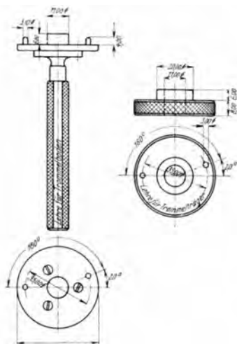
Abb. 130. Normallehre für Trommel.
