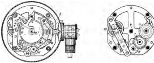
Abb. 18. Schema eines zwangsläufigen Drehzahlmessers Bruhn.
