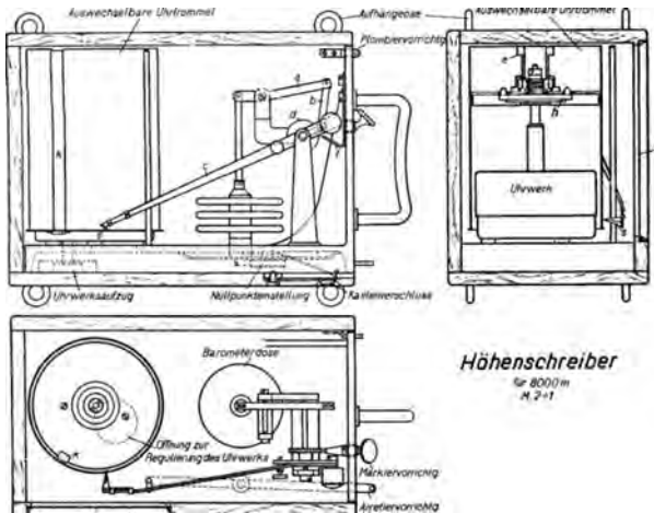
Abb. 106. Schema des Normalhöhenmessers.
