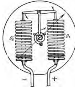
Abb. 261. Staudruck-Fahrtmesser mit Dosensätzen (A. E.-G.).
