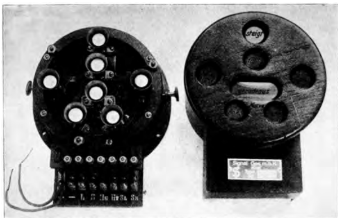
Abb. 184. Neigungsmesser nach Oppermann, Lampenanordnung („Signal“ Kiel).
