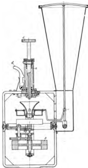
Abb. 178. Kreiselneigungsmesser (Ges. für Nautische Instrum.).
