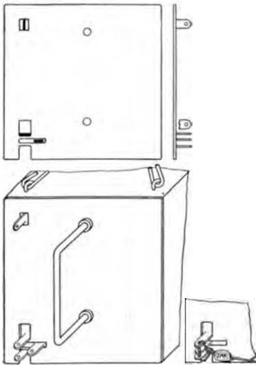
Abb. 133. Sicherung und Plombierung,
