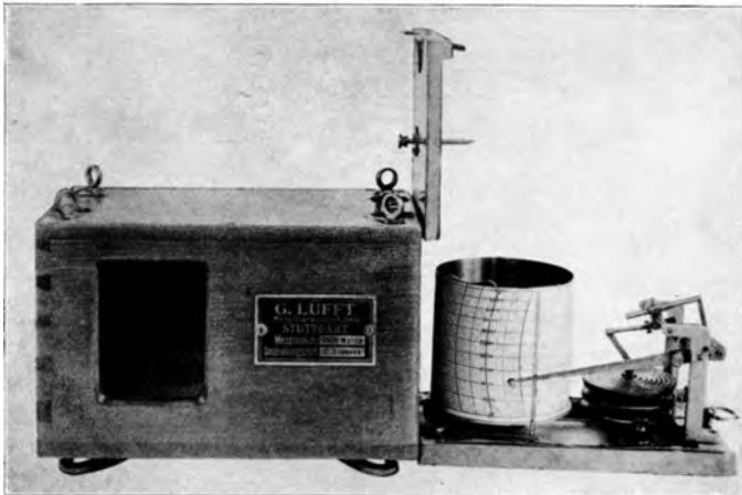
Abb. 122. Höhengreiber (Lufft).
