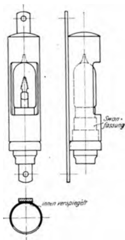
Abb. 293. Positionslicht.
