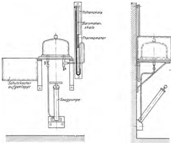
Abb. 151. Einzelprüfstand für Höhenmesser (Jahn).
