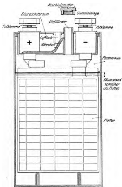
Abb. 277. Akkumulator (Varta).
