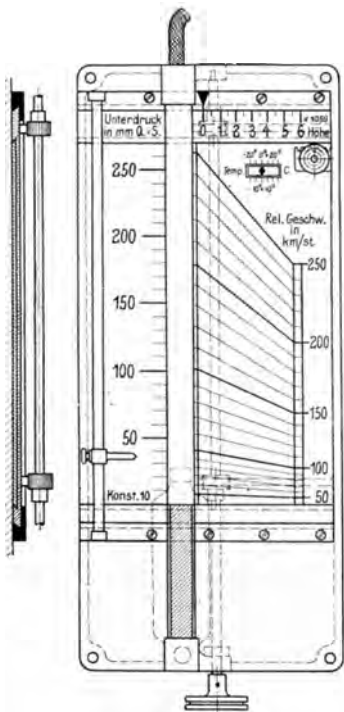
Abb. 267. Staudruck-Fahrtmesser mit Höhen- und Temperaturkorrektur (Bruhn).
