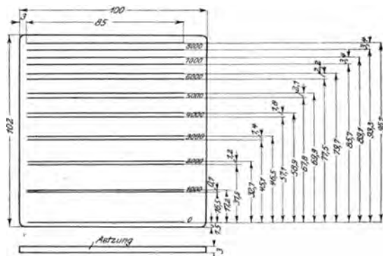
Abb. 149. Toleranzlehre für Höhenschreiberdiagramme (Goerz).
