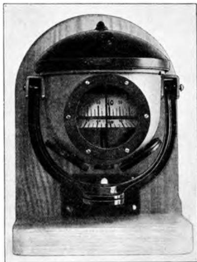
Abb. 215. Trommelkompaß (Ludolph) nach Dr. Neuber.
