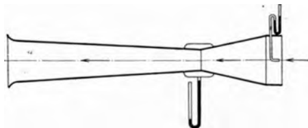
Abb. 252. Einfach-Saugrohr (Venturi).
