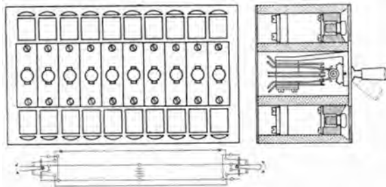
Abb. 357. Maschinentelegraph (Böker, Krüger & Co.).
