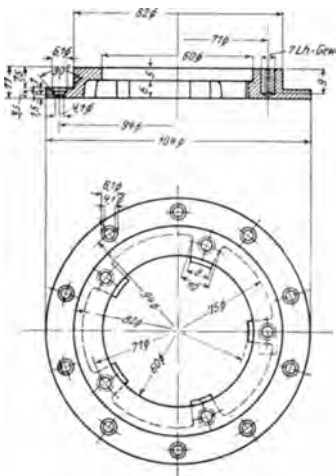
Abb. 57. Kleiner Normalflansch für Benzinuhren.
