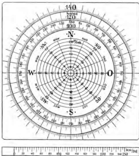
Abb. 224. Kurschieber (Wichmann).
