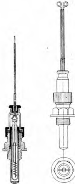
Abb. 79. Körper des Fernthermometers (Guggenheimer).
