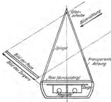
Abb. 219. Prinzip des Spiegelkompasses nach Bennewitz.
