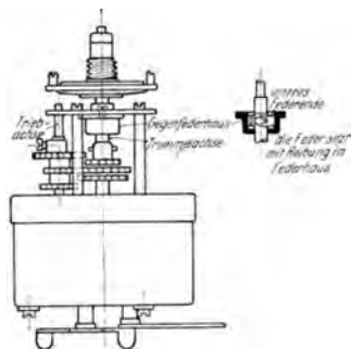
Abb. 132. Umschaltbares 2-4-6-Stundenuhrwerk.
