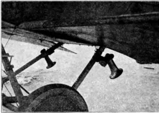
Abb. 315. Montage der Sirenen.
