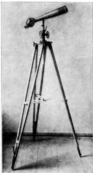
Abb. 372. Stativ des Fernrohres (Zeiß).
