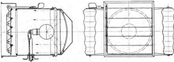
Abb. 321. Signalgerät (Alig).
