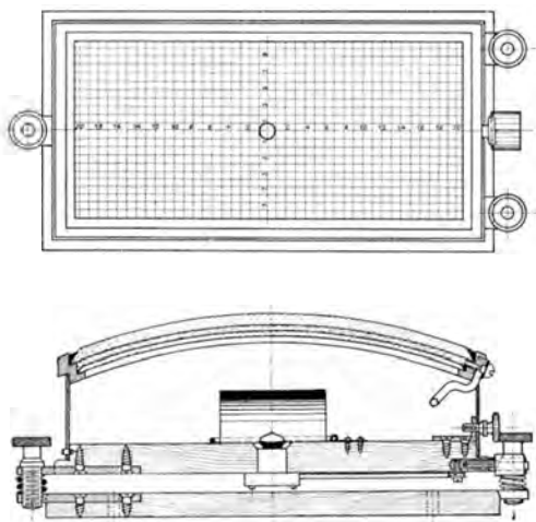
Abb. 168. Libelle für Luftschiffe (Ges. für Nautische Instrum.).
