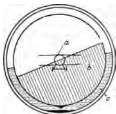
Abb. 175. Schaubild des Fliegerhorizonts (Anschütz).
