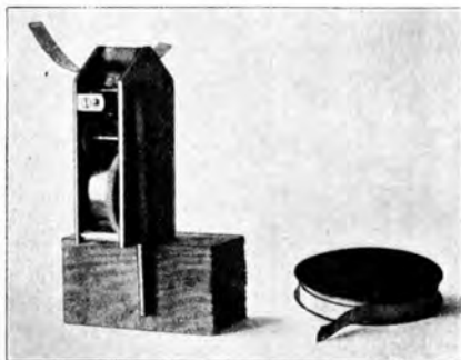
Abb. 308. Uhrwerk und Magnesiumstreifen der Magnesiumfackel (Boehm).
