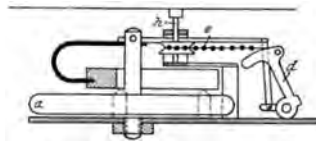
Abb. 85. Hebelwerk (Scholz).
