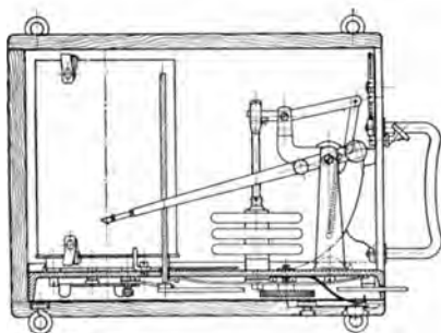
Abb. 116. Höhenschreiber (Ott).
