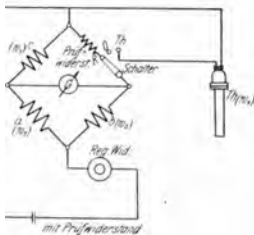
Abb. 78. Dasselbe mit Prüf-widerstand.
