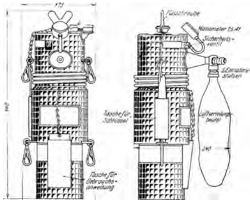
Abb. 331. Atemgerät (Ahrendt & Heylandt).
