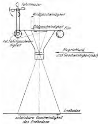
Abb. 241. Verfahren zur Windbestimmung nach Bennewitz.
