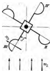
Abb. 242. Schalenkreuz.
