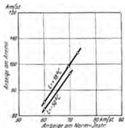
Abb. 244. Temperatureinfluß auf die Drehgeschwindigkeit.
