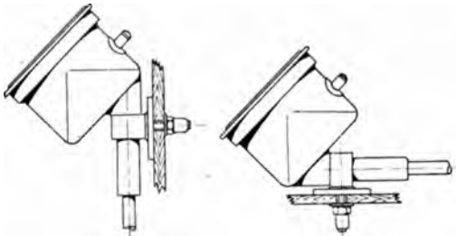
Senkrechter Antrieb.
