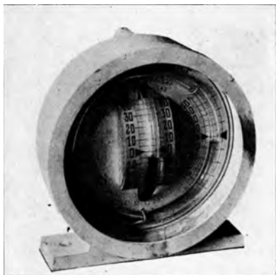
Abb. 171. Neigungsmesser „Kromer“.
