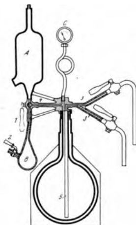
Abb. 344. Schema der Umfüllvorrichtung.
