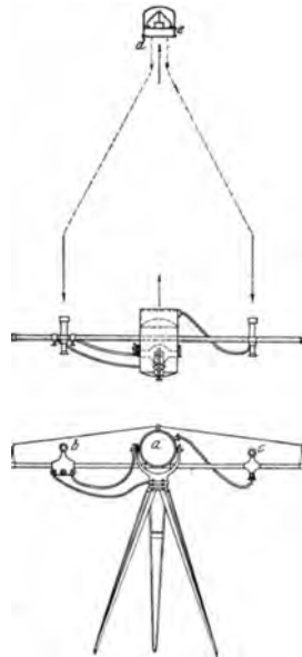
Abb. 322. Signalverfahren mit Tripelspiegel (Graß & Worff).
