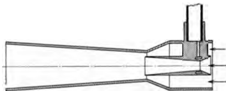
Abb. 253. Doppel-Saugrohr (Bruhn).
