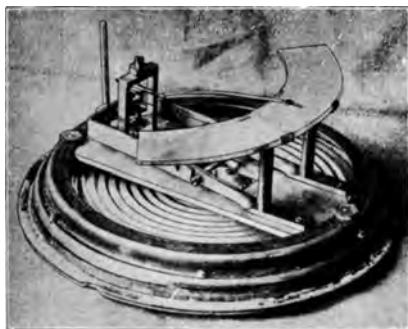
Abb. 259. Staudruck-Fahrtmesser, Manometer mit Metallmembrane (franz.).
