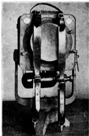
Abb. 306. Azetylscheinwerfer (Bamag).
