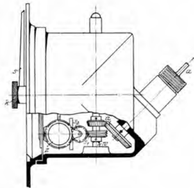
Abb. 35. Inneres des Prüfstandes (Morell).
