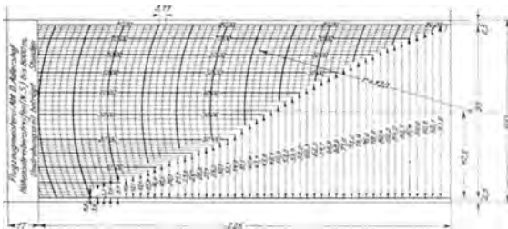
Abb. 128. Normaldiagrammstreifen für 8000 m Höhenschreiber.
