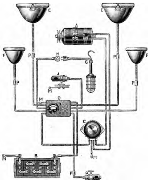
Abb. 281. Lichtenanlage nach Eisemann.
