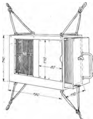
Abb. 135. Gehäuse des Höhenschreibers.
