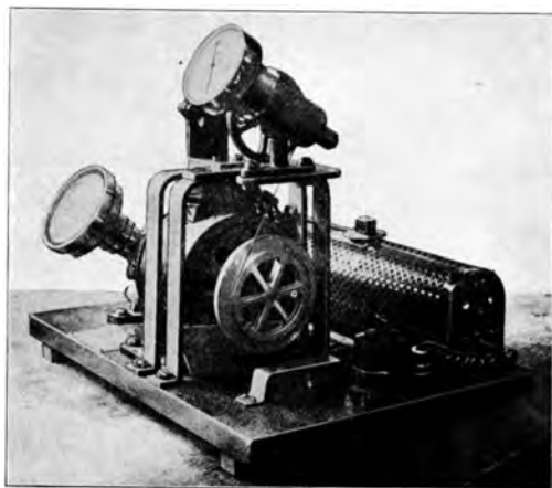
Abb. 37. Prüfstand für Drehzahlmesser (Deuta).
