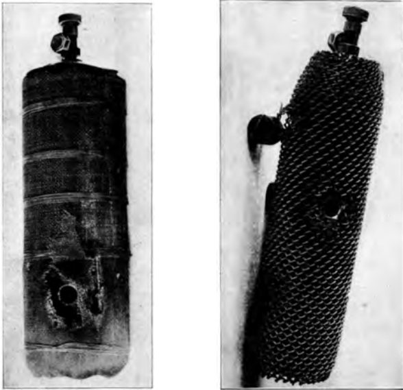
Abb. 329. Beschußversuche an Sauerstoffbomben durch gewöhnliche Munition
