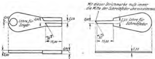
Abb. 125. Abnahmelehren für Zeiger und Schreibfeder.
