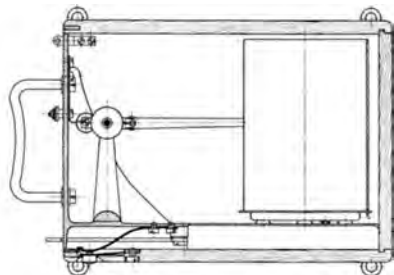
Abb. 108. Höhengschreiber (Goerz).
