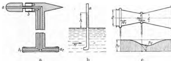
Abb. 251. a Pitotrohr, b Staurohr, c Venturirohr.
