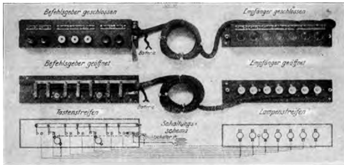
Abb. 356. Befehlsübermittler mit Lämpchen.
