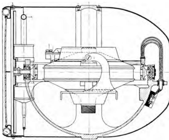
Abb. 176a. Fliegerhorizont, Seitensicht (Anschütz).
