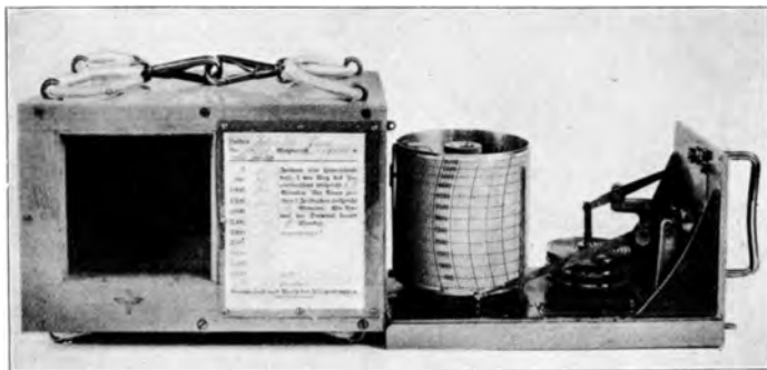
Abb. 112. Höhenschreiber (Goerz).
