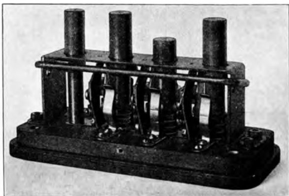
Abb. 300. Druckknopfschalter mit gemeinsamer Auslösung nach E. Franz.
