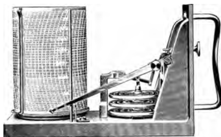
Abb. 115. Höhenschreiberwerk (Scholz).
