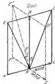
Abb. 231. Abtriftwinkel und Vorhaltwinkel.
