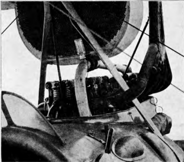
Abb. 71. Einbau des Kühlwasserthermometers.
