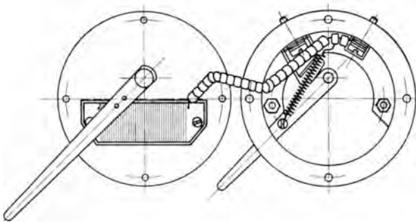
Abb. 299. Schalter (Ruhstrat.).
