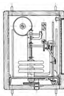
Abb. 118. Höhenschreiber (Ott).
