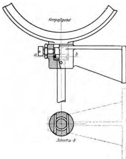
Abb. 207. Gabelbefestigung (Bamberg).
