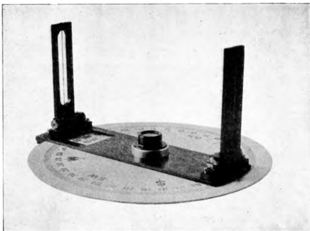
Abb. 233. Peilscheibe (Bamberg).
