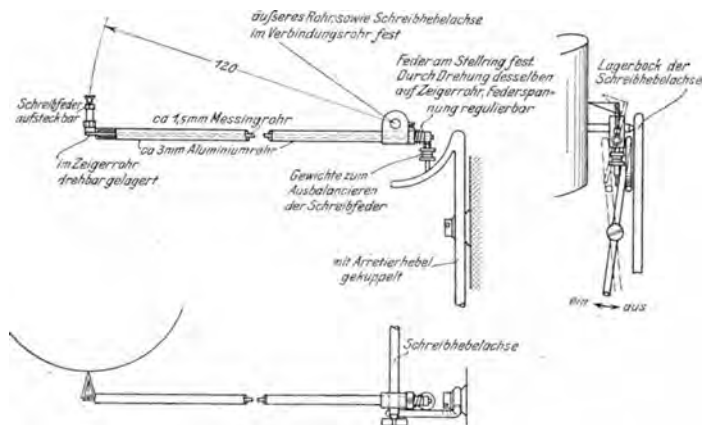
Abb. 126. Lageunempfindlicher Schreibhebel.
