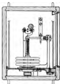
Abb. 110. Höhenschreiber (Goerz).
