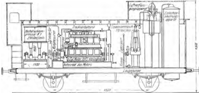
Abb. 346. Luftverflüssigungsanlage im Eisenbahnwagen (Ahrendt & Heylandt).
