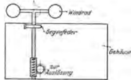
Abb. 134. Selbsttätige Schaltung für Höhenschreiber.
