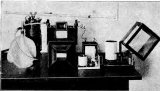
Abb. 347. Eichung von Atemgeräten in der pneumatischen Kammer (Gasuhr, Höhenschreiber, Chronograph).
