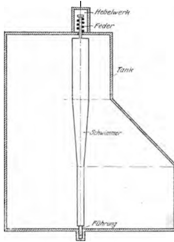
Abb. 46. Druckschwimmer nach Lachmann.
