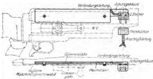
Abb. 352. Maschinengewehrheizung.
