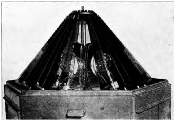
Abb. 305. Signalisierung durch Leuchtfleur (Alig). (Farbgläser geöffnet.)
