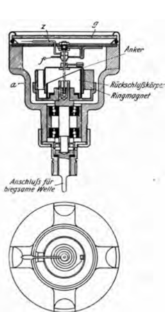
Abb. 9. Schema eines Wirbelstromdrehzahlmessers (Deuta).
