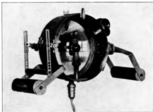
Abb. 317. Signalgerät (Zeiss).
