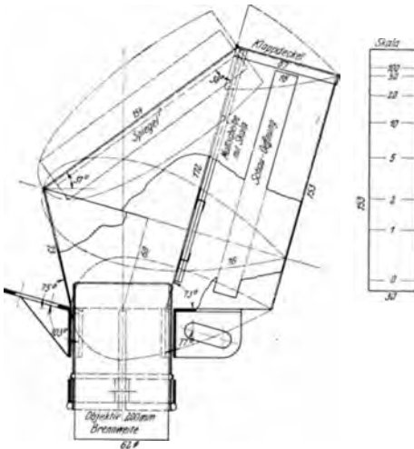
Abb. 153. Landungsmesser „Optika“.
