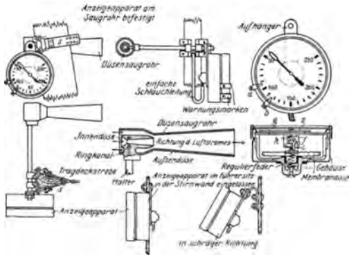
Abb. 265. Staudruck-Fahrtmesser (Bruhn).
