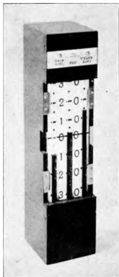
Abb. 173. Neigungsmesser nach Dr. Neuber.
