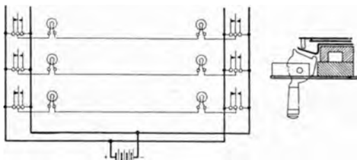
Abb. 358. Befehlsübermittler mit Gegenruf (Arnheim).
