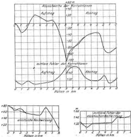
Abb. 148. Prüfergebnis eines Höhenschreibers (Ott).
