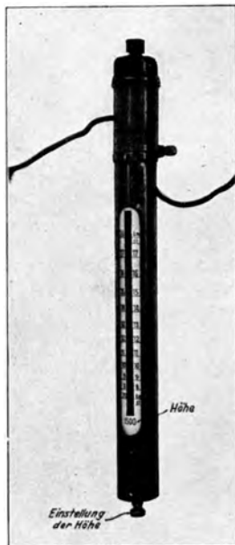
Abb. 268. Staudruck-Fahrtmesser mit Höhenkorrektur nach Dr. Neuber.
