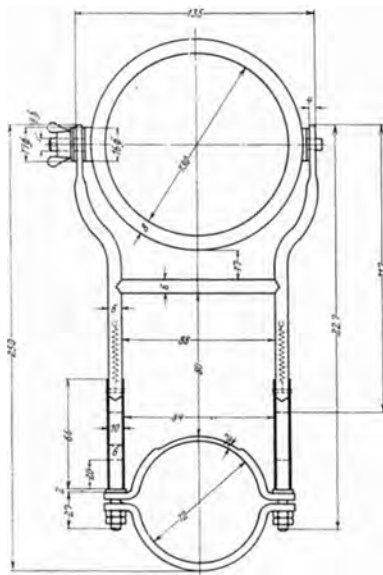
Abb. 361. Maschinengewehrspiegel nach Oppermann ((Bernheim).
