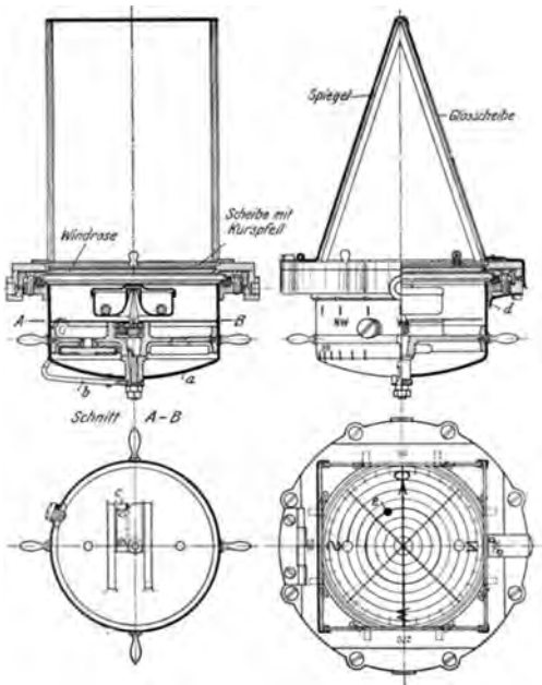
Abb. 229. Reisekompaß nach Bennewitz (Bamberg).
