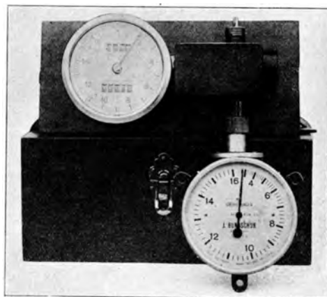
Abb. 36. Universalprüfstand Bruhn.
