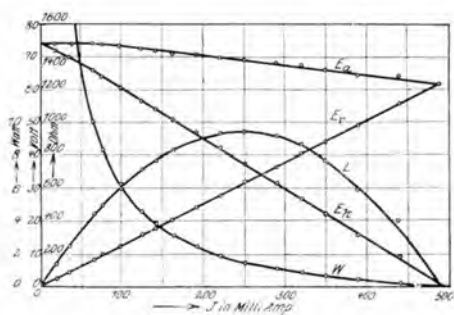
Abb. 26. Charakteristik des Fern-drehzahlmessers (Morell). (Nach Dr. Wilke.)
