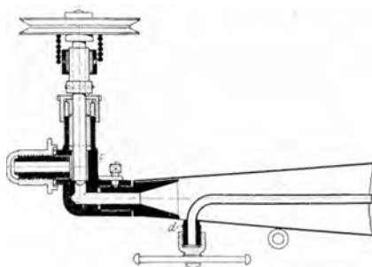
Abb. 325. Signalgerät „Möve“.
