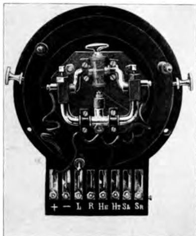
Abb. 183. Neigungsmesser nach Oppermann; U-Rohr („Signal“ Kiel).
