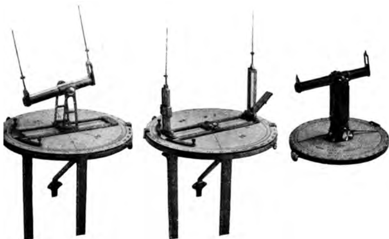
Abb. 235. Peilscheiben (Ludolph).
