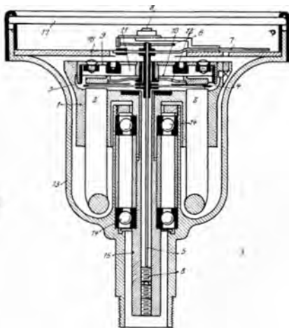
Abb. 10. Schema eines Wirbelstromdrehzahlmessers (Ihle).
