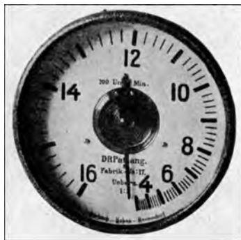
Abb. 13. Drehzahlmesser (Lehmbek),
