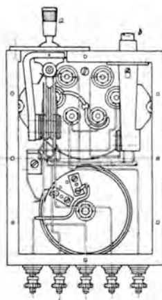
Abb. 81. Fernthermometer (Guggenheimer).
