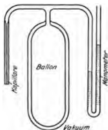
Abb. 157. Schema des Variometers „Bestelmeier“.
