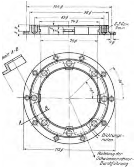
Abb. 56. Großer Normalflansch für Benzinuhren.
