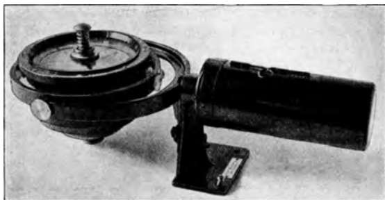
Abb. 191. Rumpfkompas, sog. Marine-Leuchtkompas (Bamberg).
