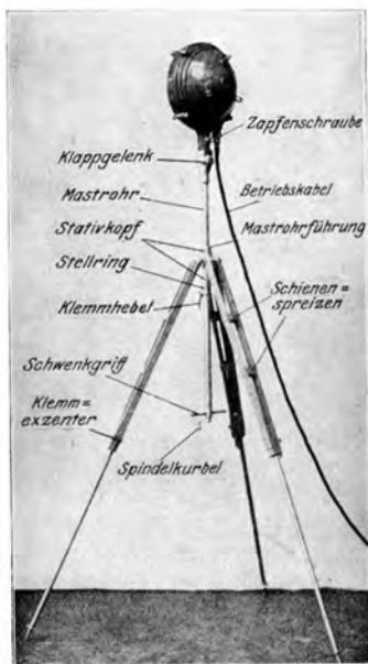
Abb. 310. Wiskottscheinwerfer (Busch).
