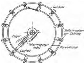
Abb. 43. Schema einer Benzinuhr mit linearer Teilung (Franz).
