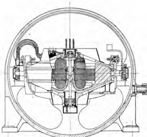
Abb. 176c. Fliegerhorizont, Querschnitt (Anschnitt).
