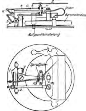
Abb. 83 u. 84. Normales Hebelwerk des Höhenmessers.
