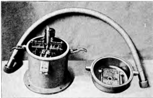
Abb. 21. Fern-drehzahlmesser (Morell). Geber.
