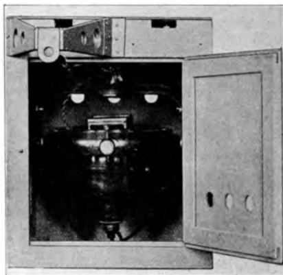
Abb. 220f. Selenkoinpaß, Gehäuse (Bamberg).
