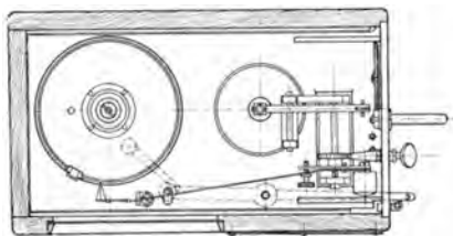
Abb. 117. Höhenschreiber (Ott).
