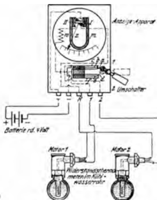
Abb. 75. Schaltschema des Fernthermometers Hartmann & Braun.
