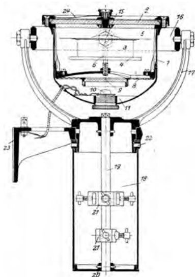
Abb. 204. Normalisierter Rumpfkompas.
