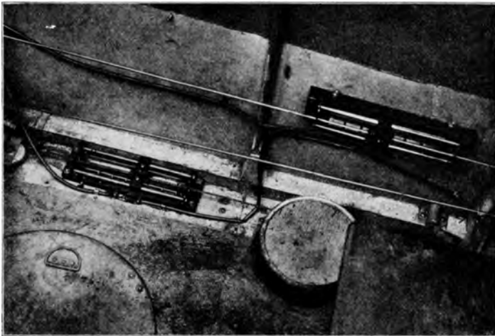
Abb. 182. Neigungsmesser nach Oppermann; Seitensteuerkontakte („Signal“ Kiel).
