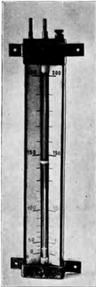
Abb. 260. Staudruck-Fahrtmesser mit Flüssigkeitsmanometer,
