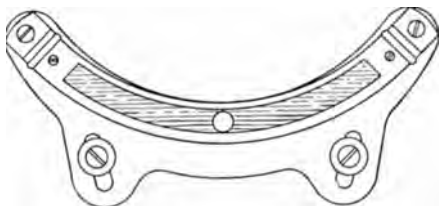
Abb. 166. Neigungsmesser (Fueß).
