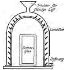
Abb. 146. Thermorezipient (Fueß).
