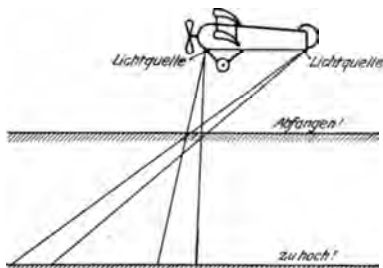
Abb. 154. Optischer Landungsmesser nach Bennewitz.
