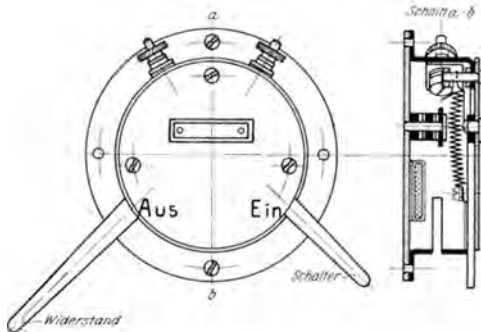
Abb. 298. Beleuchtungsschalter (Ruhstrat.).
