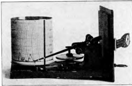
Abb. 121. Höhengreiberwerk (Fuess).
