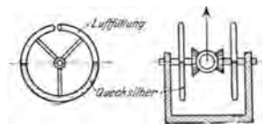
Abb. 142 und 143. Dichtemessung nach Dr. Blasius.
