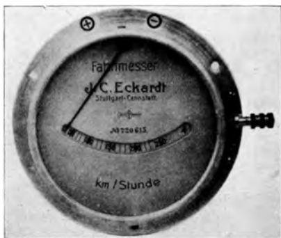
Abb. 269. Staudruck-Fahrtmesser mit Höhenkorrektion (Eckardt).
