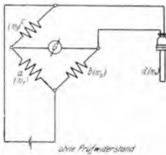
Abb. 77. Schaltschema des Thermometers (Guggenheimer).
