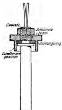
Abb. 72. Körper des Dampfdruckthermometers (Atmos).
