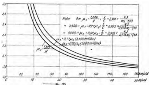
Abb. 243. Relative Drehgeschwindigkeit (c) in Abhängigkeit von der Windgeschwindigkeit (nach Dr. Wilke) und Dichte (u).
