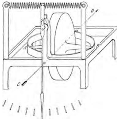
Abb. 170. Prinzip des Steuerzeigers (Drexler).
