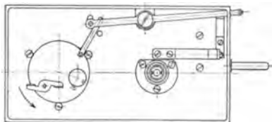
Abb. 111. Höhenschreiber (Goerz).
