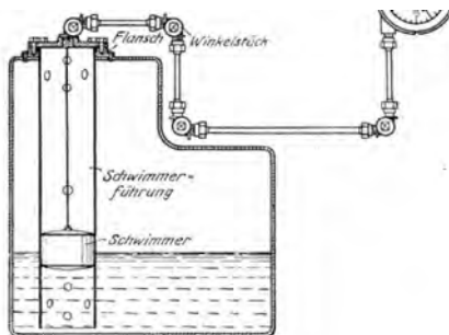
Abb. 39. Schema einer Benzinuhr mit Schwimmer (Morell).
