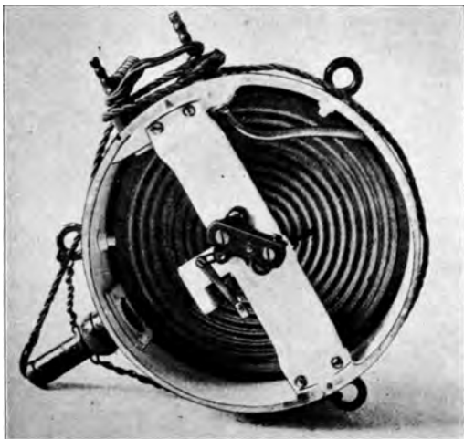
Abb. 258. Staudruck-Fahrtmesser, Manometer mit Metallmembrane (Eckardt).
