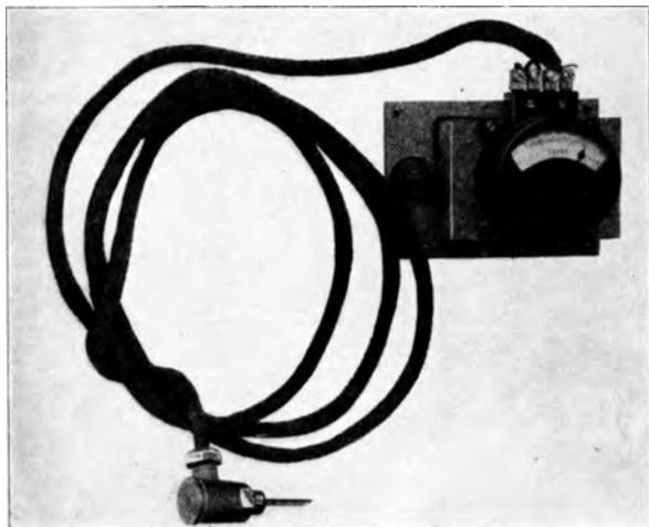
Abb 76. Fernthermometer (Hartmann & Braun).
