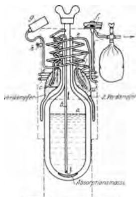
Abb. 330. Schema eines Atemgeräts mit flüssiger Luft (Ahrendt & Heylandt)
