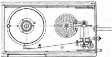
Abb. 109. Höhenschreiber (Goerz).
