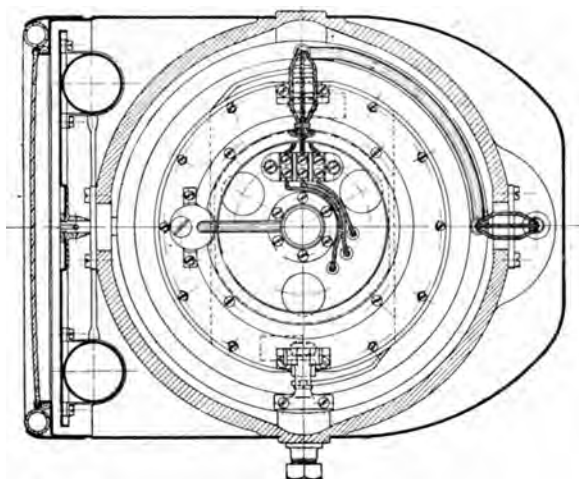
Abb. 176b. Fliegerhorizont, Aufsicht (Anschütz).
