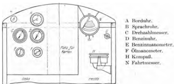
Abb. 386. Normaleinbau in Marinetfugzeugen.
