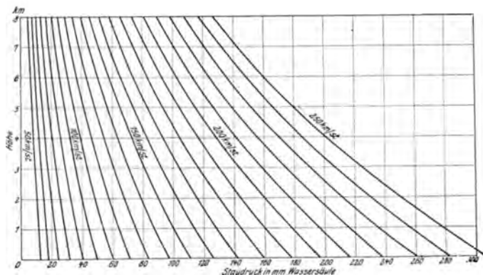
Abb. 273. Staudruckkurven.
