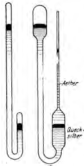
Abb. 275 und 276. Beschleunigungsmesser nach Bennewitz.
