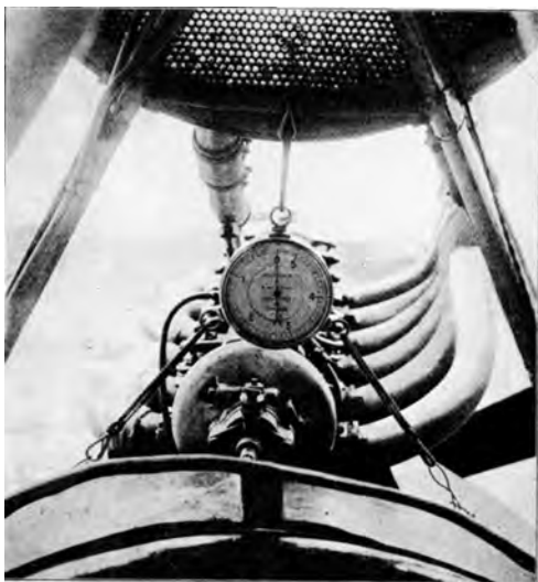
Abb. 102. Aufhängung mittels Gummischnüre eines Höhenmessers.
