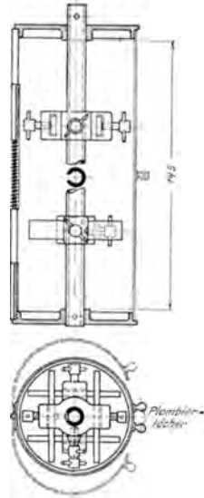
Abb. 208. Normalisierte Kompensierungsvorrichtung
