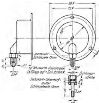
Abb. 59. Normalien für Manometer (Benzin und Öl).
