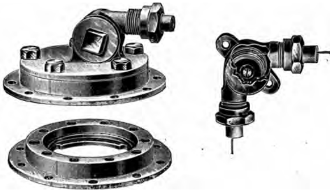
Abb. 54. Benzinuhrflansch Maximall.
