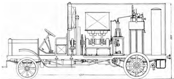
Abb. 345. Luftverflüssigungsanlage auf Kraftwagen (Ahrendt & Heylandt).
