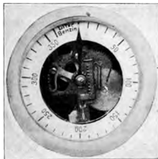
Abb. 44. Benzinuhr (Franz).
