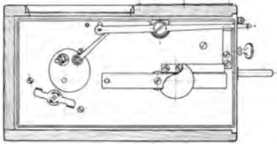
Abb. 120. Höhengreiber (Ott).
