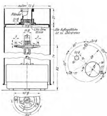
Abb. 129. Normalien der Höhenschreibertrommel.
