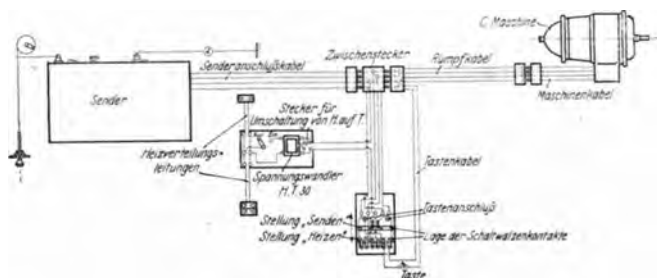
Abb. 348. Schaltskizze des F. T.-Generators für Heizzwecke.
