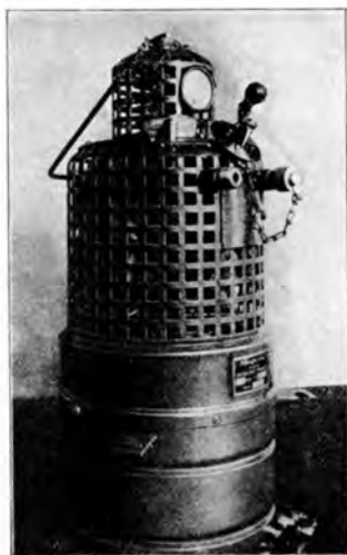
Abb. 338. Atemgerät, große Form („Flüssige Gase“, Kiel).
