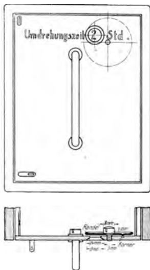
Abb. 136. Umdrehungszeitanzeiger.
