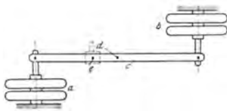
Abb. 101. Schema einer nachwirkungsfreien Dosenanordnung.
