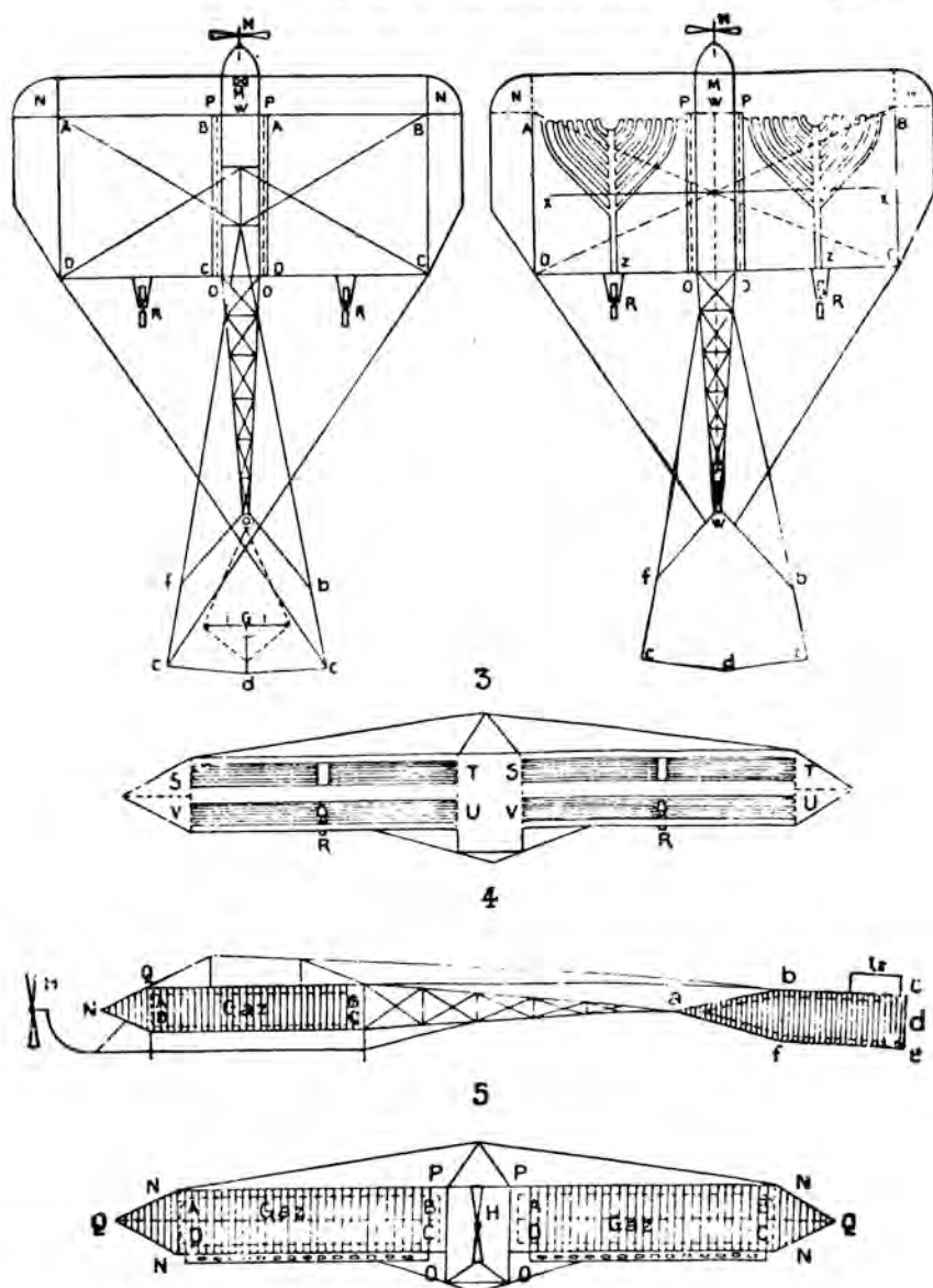
FIG. 140. — Statoplane BOCAUYVA.
