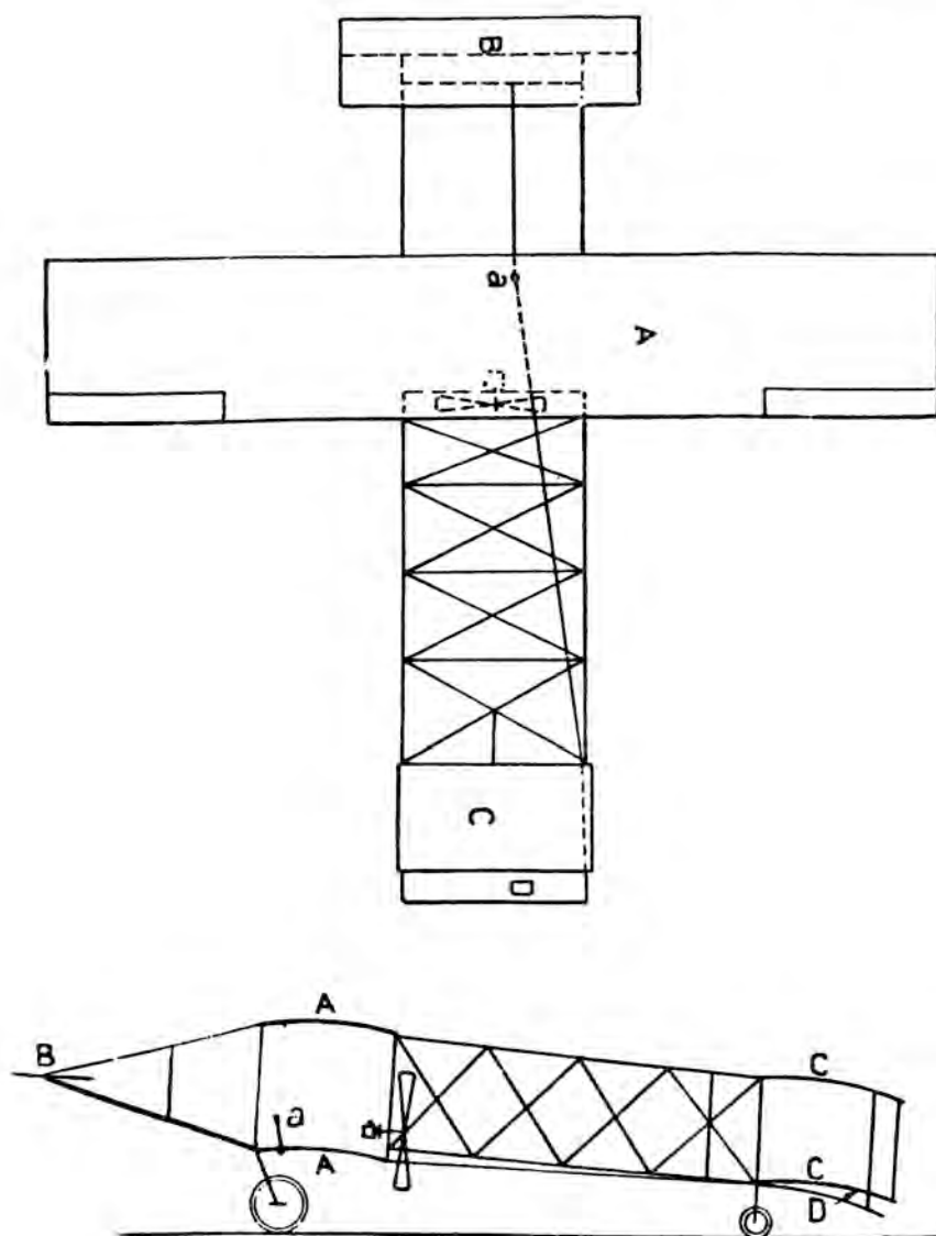
FIG. 142 et 143. — Biplan GOUPEY ET VOISIN.
