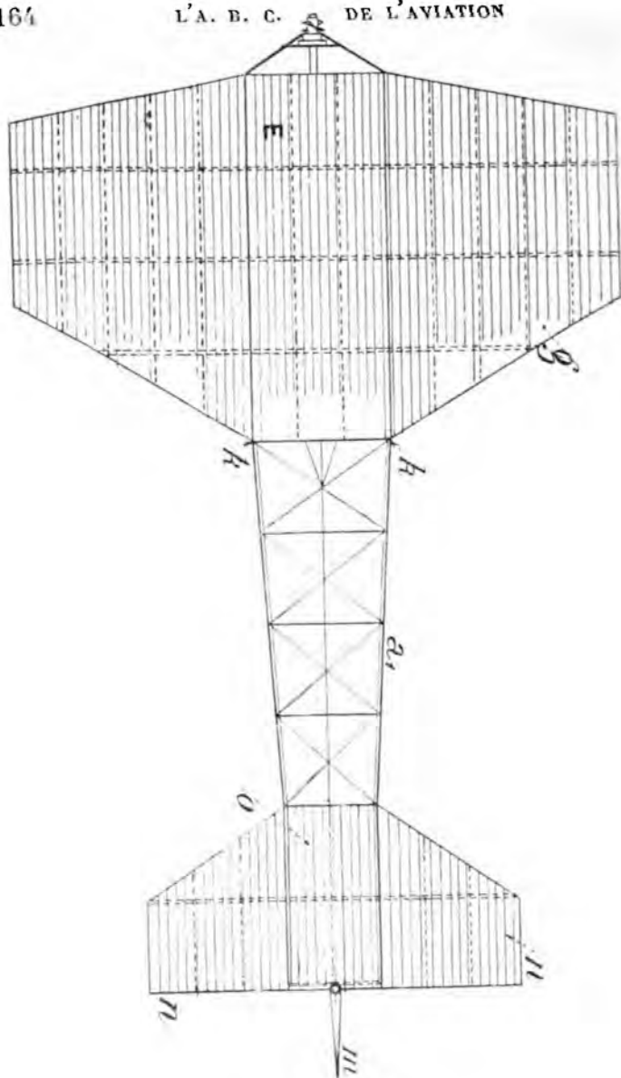
FIG. 118 Monoplan PUISEUX (plan).
