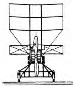
FIG. 130 Multiplan Hayot (vu de face).
