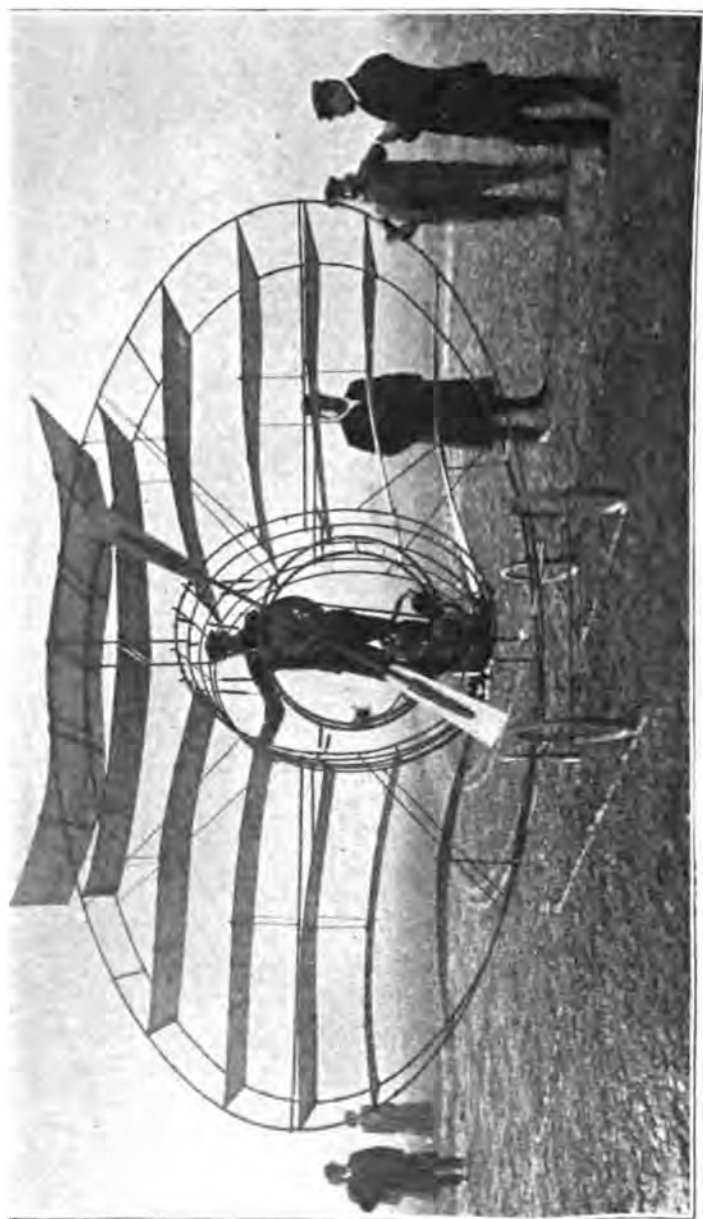
FIG. 131 Multiplan du Marquis d'ERQUEVILLY.
